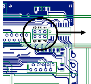
Fig. [20.1] CAMBIO de LÓGICA CN2 CN2 tipo entrada PNP J1 (2-3) y J2 (5-6) NPN J1 (1-2) y J2 (4-5)
