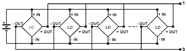
CONEXIÓN DE 4 CÉLULAS O MÁS EN PARALELO
