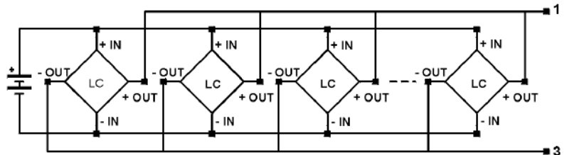
RACCORDEMENT 4 CELLULES OU PLUS EN PARALLELE
