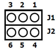
Fig. [20.1] CAMBIO de LÓGICA CN2 CN2 tipo entrada PNP J1 (2-3) y J2 (5-6) NPN J1 (1-2) y J2 (4-5)
