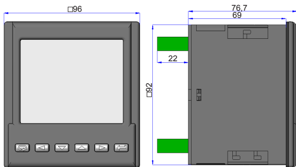
Fig. 2. Meter dimensions.
